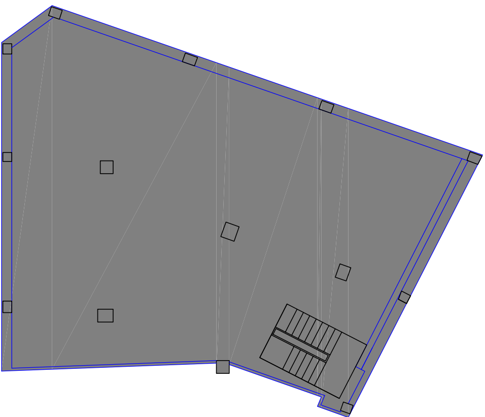
PLANTA SOTANO -1: 201,59m 2
